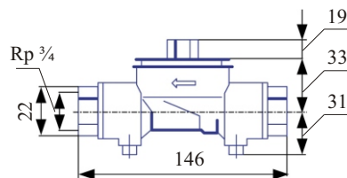
Рис.3 EAS с шаровыми кранами
